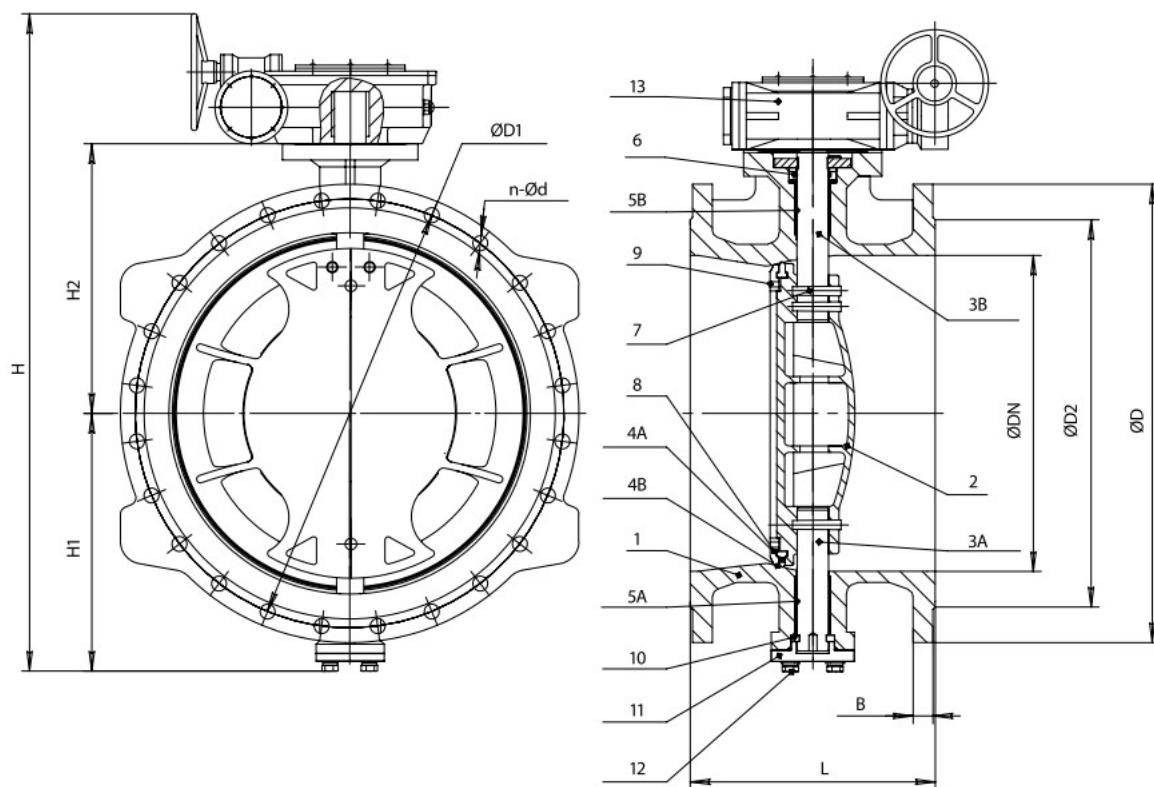
Рисунок 2. Затворы DN 700-2000
