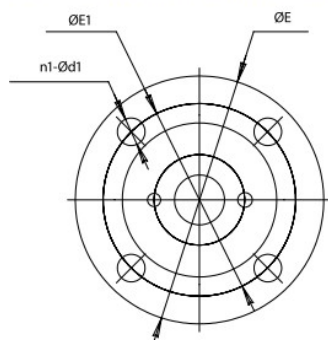
Фланец исполнительного механизма
