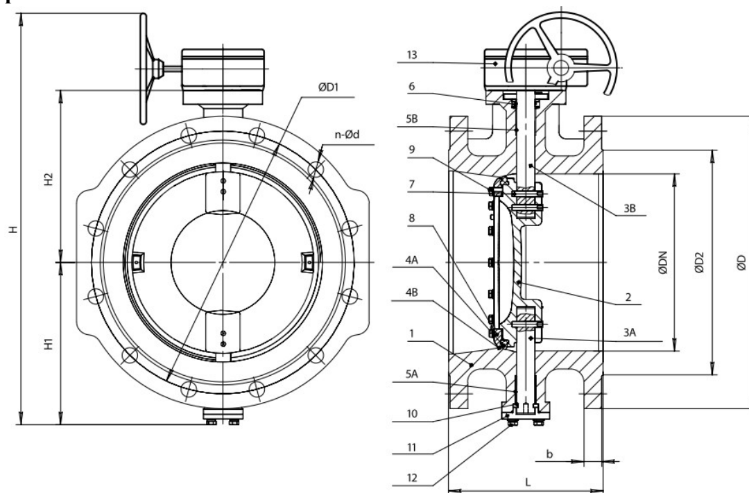
Рисунок 1. Затворы DN 300-600
