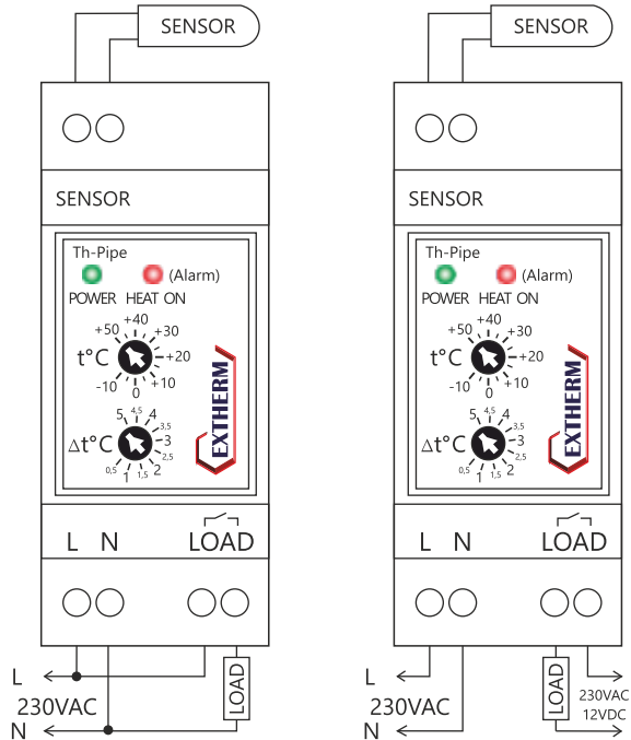
Схема подключения
