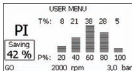
Figura 17: Vizualizarea histogramei de putere
