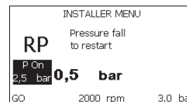
Kuva 18: Uudelleenkäynnistyspaineen asetus
