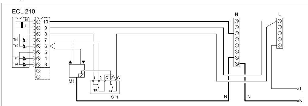
Контур системы ГВС
